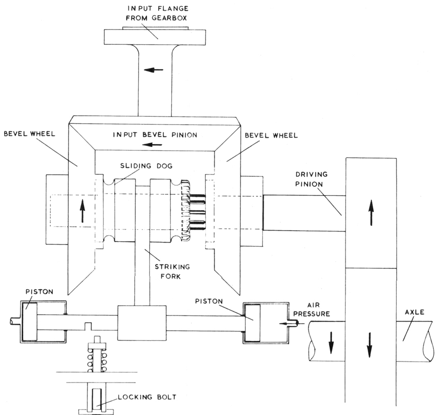
R.F. 28. FINAL DRIVE
